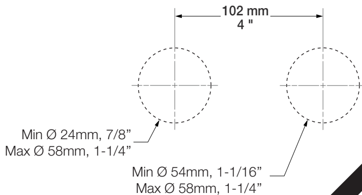
Gabarit de perçage / Hole template
